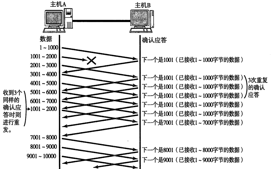
图 6.18 高速重发控制 (Fast Retransmission)
