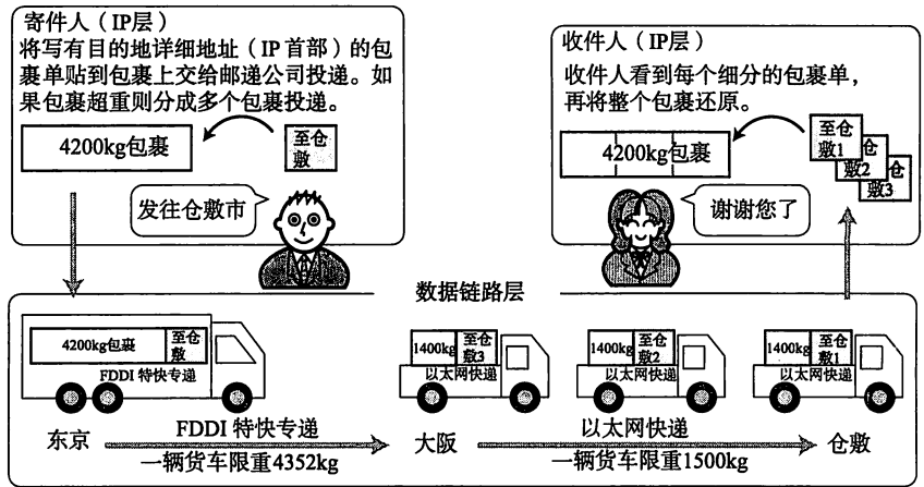
图 4.3 不同数据链路的最大传输单位
